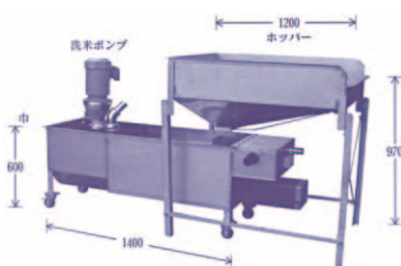
改良型洗米機 (縮尺15.7/1000)
